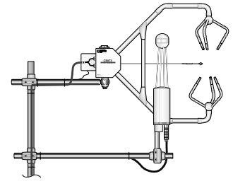
CSAT3 and CS7500
